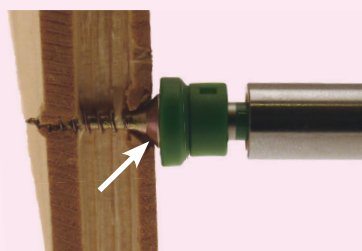
Vis en contact de la butée
